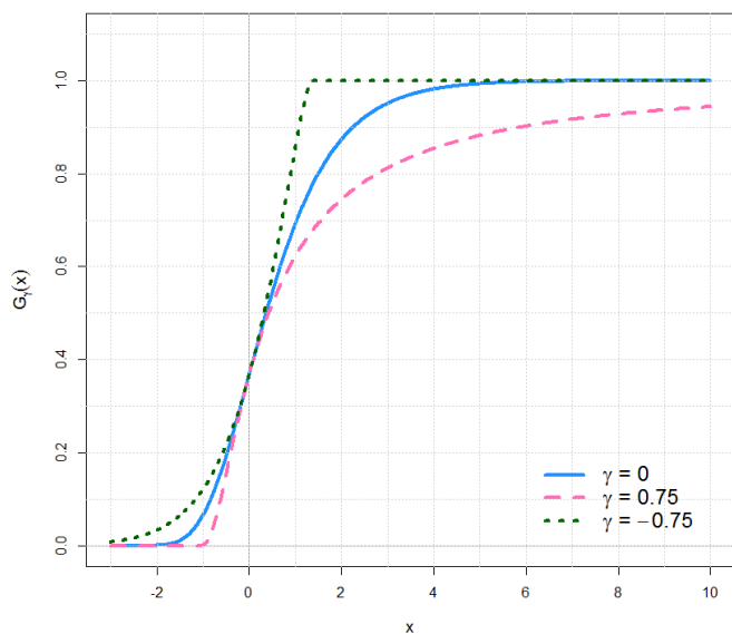
Графици функција расподеле стандардних генералисаних расподела екстремних вредности
