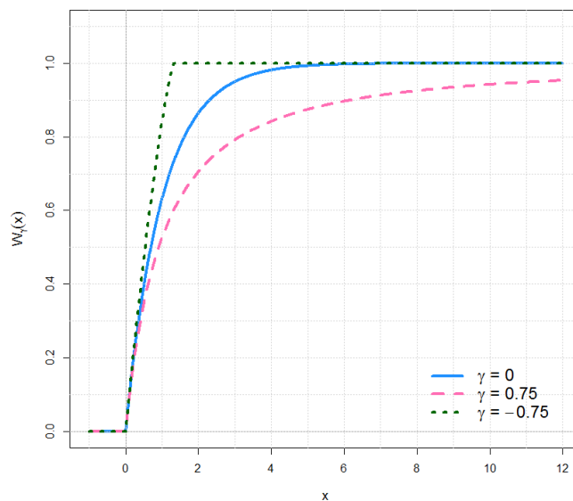
Графици функција расподеле стандардних генералисаних Паретових расподела
