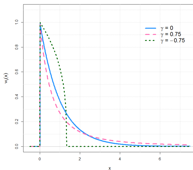
Графици густина расподеле стандардних генералисаних Паретових расподела
