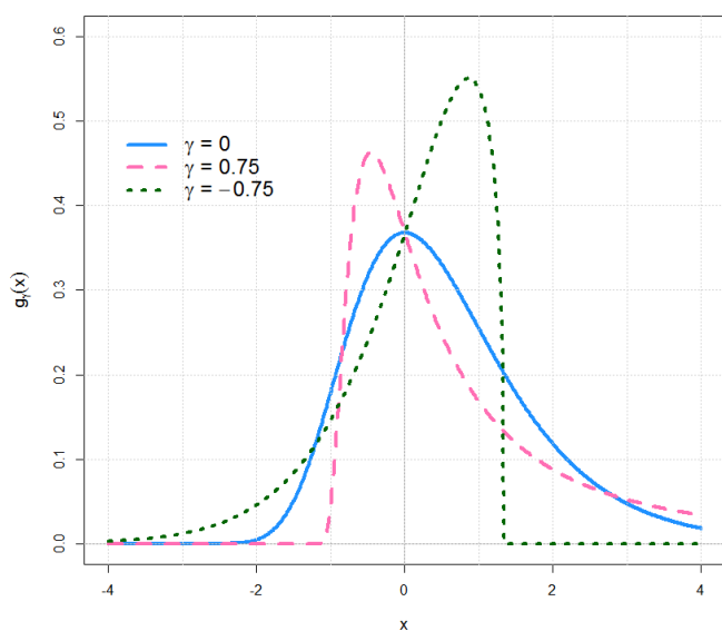
Графици густина расподеле стандардних генералисаних расподела екстремних вредности
